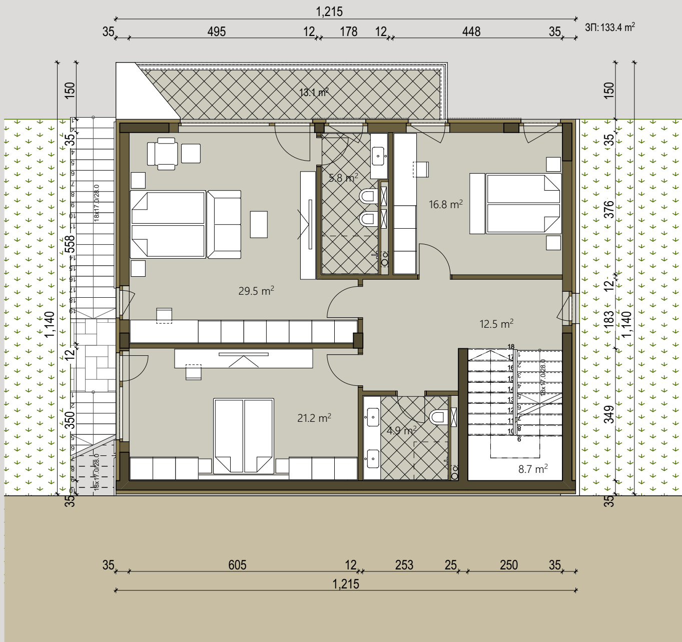
К2 РАЗПРЕДЕЛЕНИЕ - КОТА +3.05
